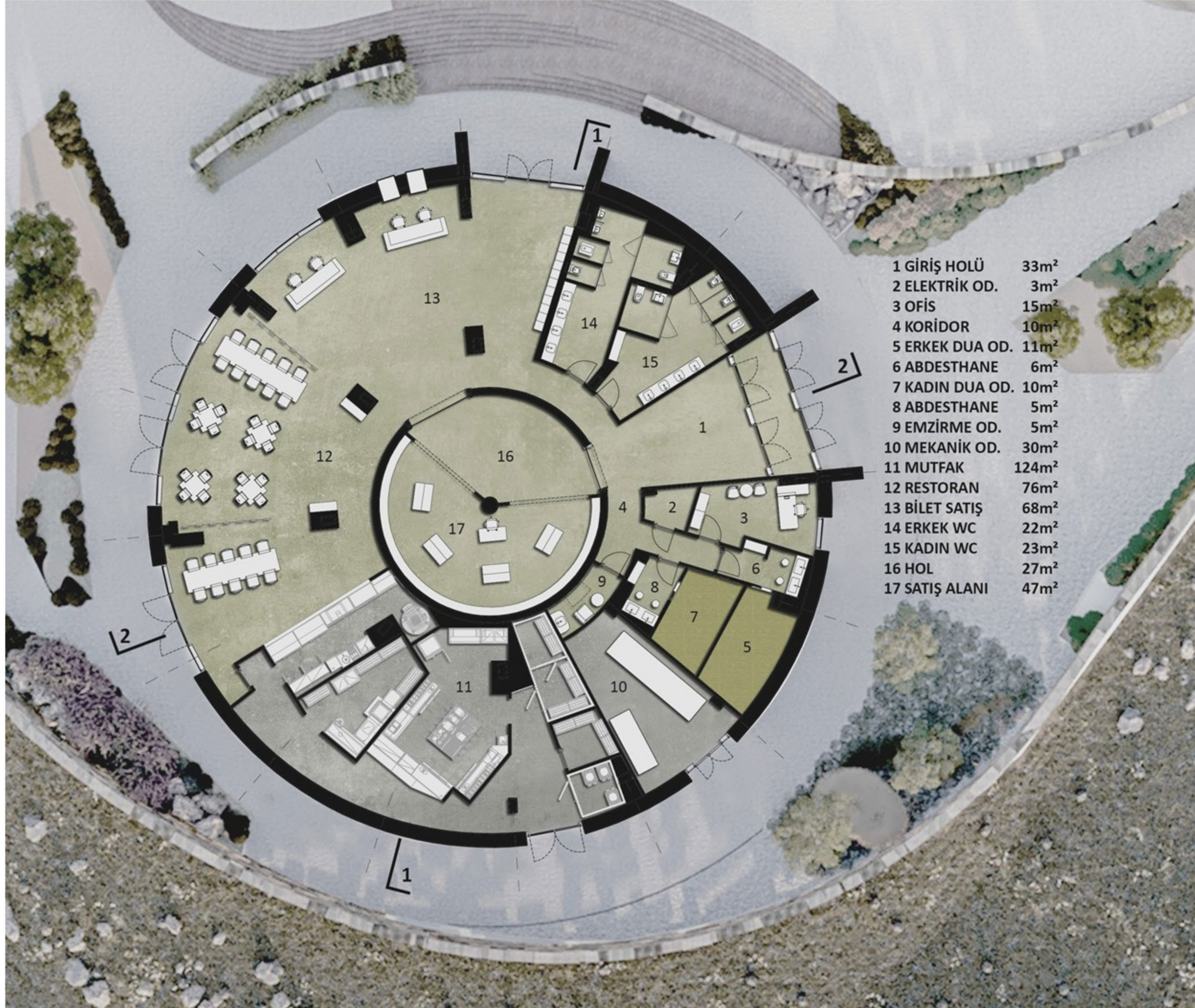
Ziyaretçi Merkezi Planı
