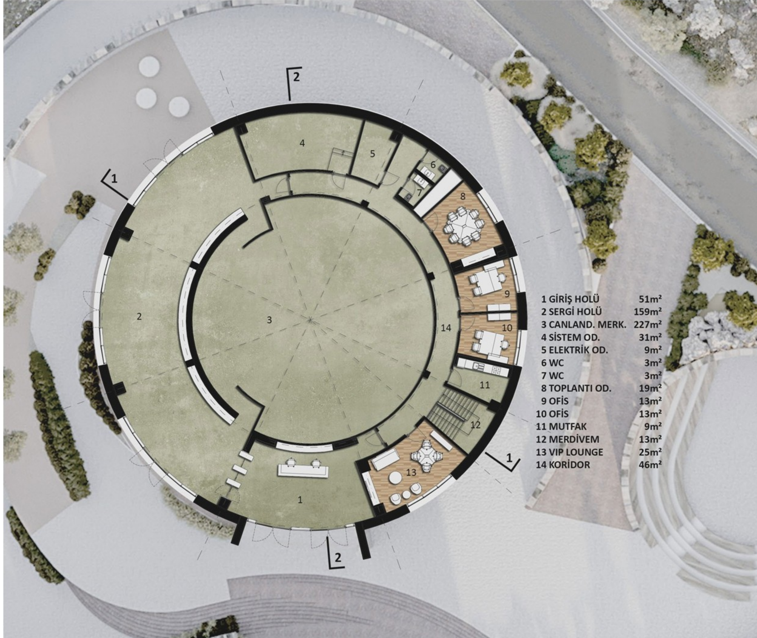
Sergileme Merkezi Planı
